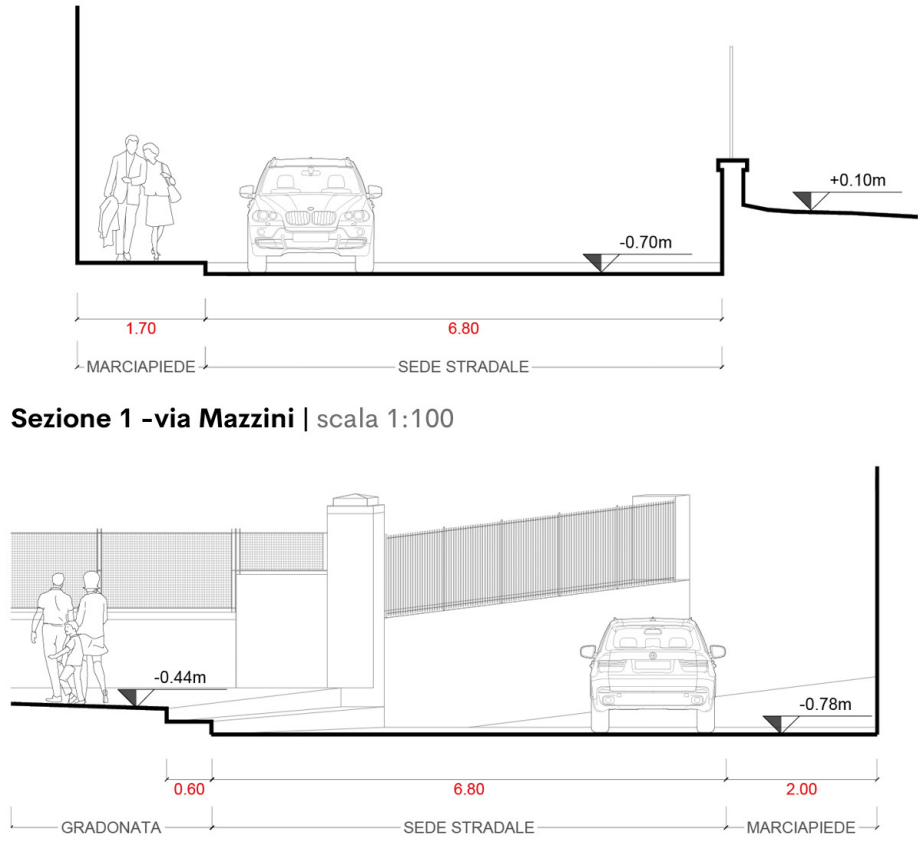
Sezione 1 -via Mazzini | scala 1:100
