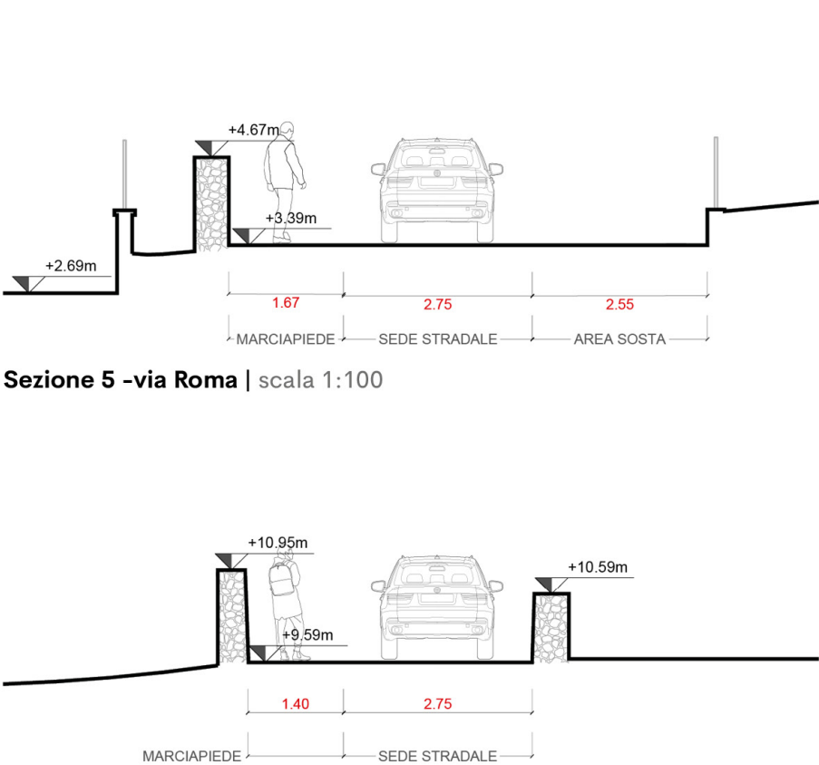
Sezione 5 -via Roma | scala 1:100
