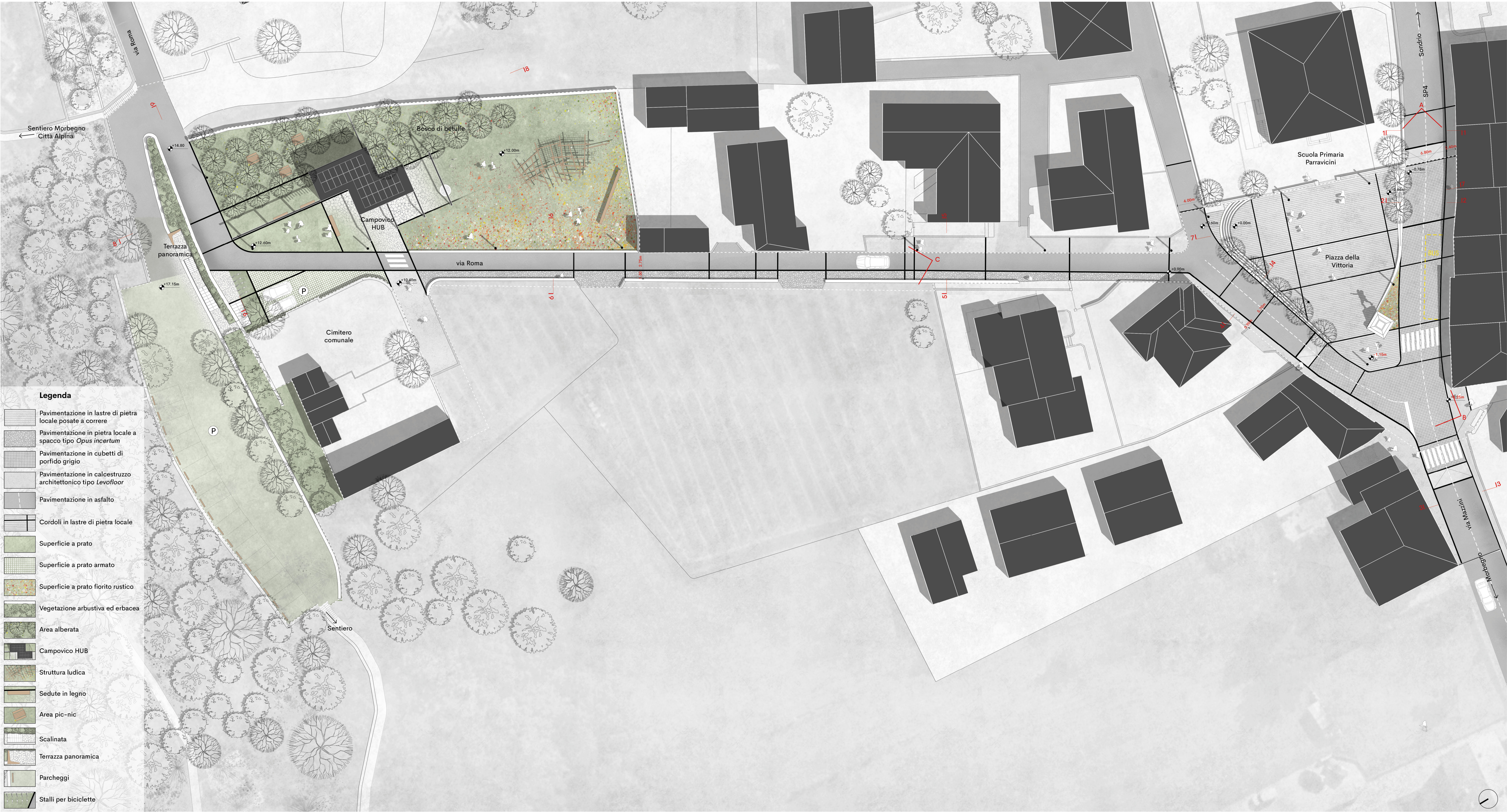
Planimetria | scala 1:300
