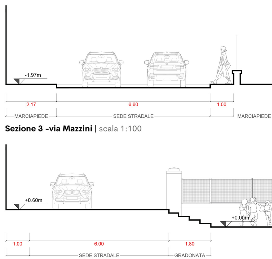
Sezione 3 -via Mazzini | scala 1:100
